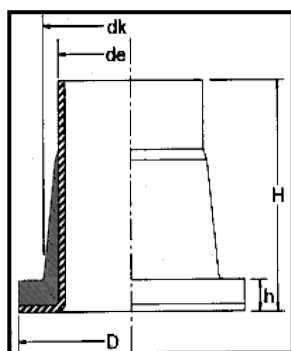
PP/LM KAULUKSET
