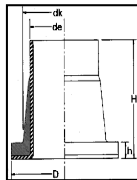
PE100/LM KAULUKSET
