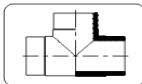
PP T-HAARA
