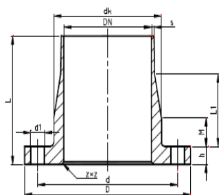
VEN KIINTOLAIPPA PN 16 LAMINOITU LIITOS
