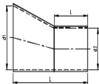
VEN SUPISTUS EPÄKESK. PN 6 LAMINOITU LIITOS
