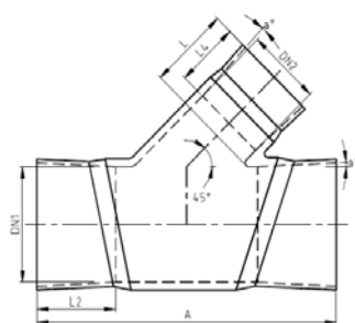
VEN T-KAPPALE 45° PN 16 LAMINOITU LIITOS
