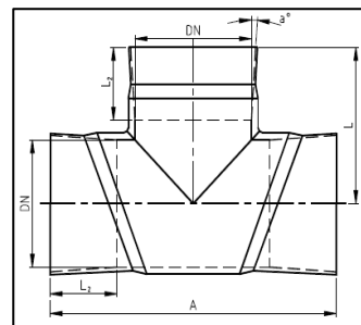
T-KAPPALE 90°
