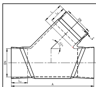
T-KAPPALE 45°
