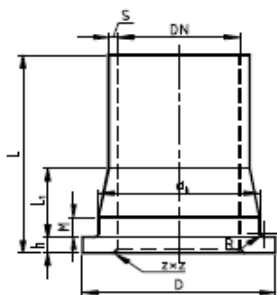
VE KAULUS PN 16 LAMINOITU LIITOS
