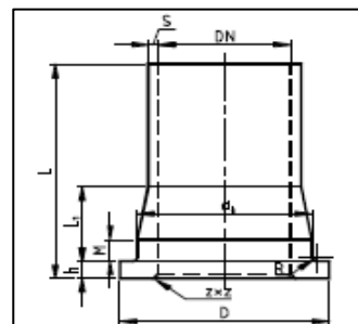
KAULUS
