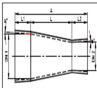
SUPISTUS KESKEINEN
