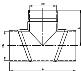
VE T-KAPPALE 90° PN 16 LAMINOITU LIITOS
