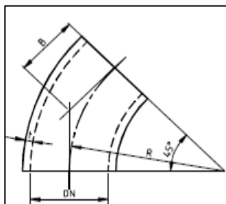
KÄYRÄ 45°
