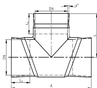
VEN T-KAPPALE 90° PN 10 MUHVILIITOS
