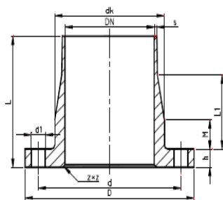
VE KIINTOLAIPPA PN 6 LAMINOITU LIITOS
