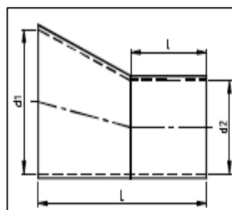
SUPISTAJA EPÄKESKEINEN
