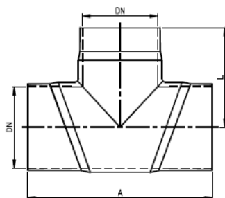
VEN T-KAPPALE 90° PN 6 LAMINOITU LIITOS
