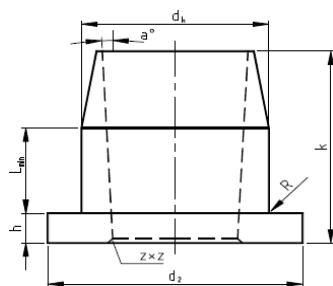
VE KAULUS PN 10 MUHVILIITOS
