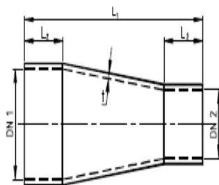
VE SUP.KESK. PN 16 LAMINOITU LIITOS
