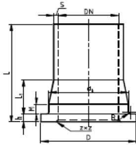
VEN KAULUS PN 16 LAMINOITU LIITOS
