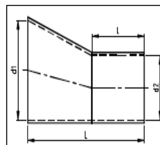
SUPISTAJA EPÄKESKEINEN
