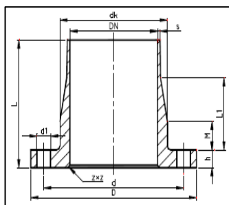
KIINTOLAIPPA
