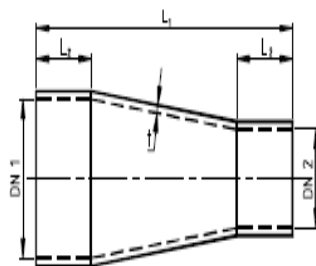
VEN SUPISTUS KESKEINEN PN 10 LAMINOITU LIITOS
