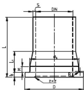
VE KAULUS PN 10 LAMINOITU LIITOS
