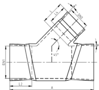
VE T-KAPPALE 45° PN 6 LAMINOITU LIITOS
