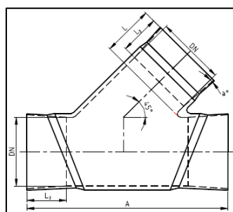
T-KAPPALE 45°
