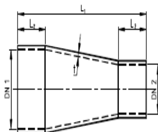
VEN SUPISTUS KESKEINEN PN 16 LAMINOITU LIITOS
