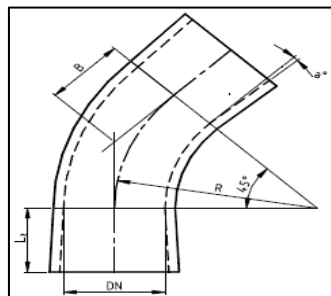
KÄYRÄ 45°
