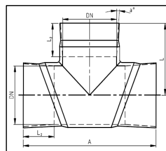
T-KAPPALE 90°
