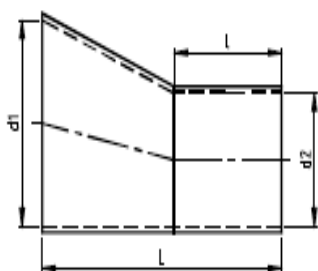
VEN SUPISTUS EPÄKESK. PN 1 LAMINOITU LIITOS
