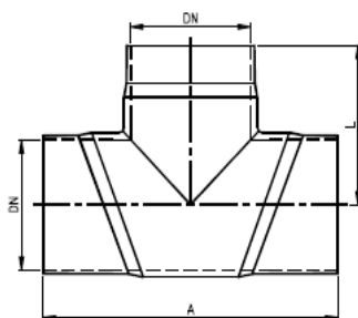
VE T-KAPPALE 90° PN 6 LAMINOITU LIITOS
