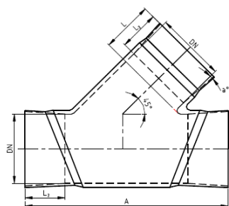
VEN T-KAPPALE 45° PN 10 MUHVILIITOS
