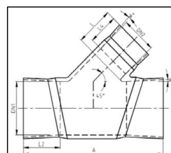
T-KAPPALE 45°
