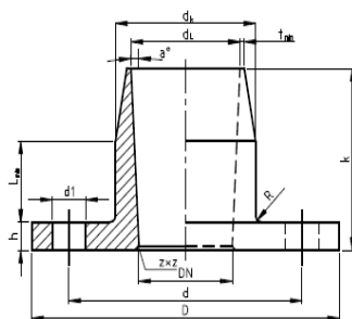
VEN KIINTOLAIPPA PN 10 MUHVILIITOS
