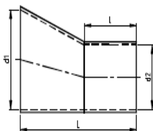
VE SUP.EPÄKESK. PN 16 LAMINOITU LIITOS
