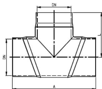
VEN T-KAPPALE 90° PN 10 LAMINOITU LIITOS
