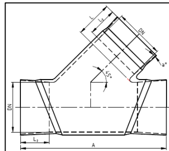
T-KAPPALE 45°
