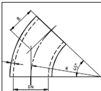
KÄYRÄ 45°
