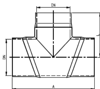
VE T-KAPPALE 90° PN 10 LAMINOITU LIITOS
