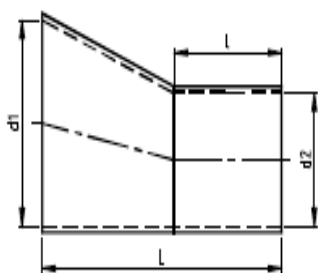
VEN SUPISTUS EPÄKESK. PN : LAMINOITU LIITOS
