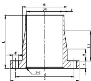
VEN KIINTOLAIPPA PN 10 LAMINOITU LIITOS
