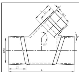
T-KAPPALE 45°
