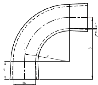
VE KAYRA 90° PN 16 MUHVILIITOS
