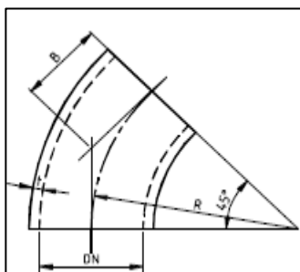
KÄYRÄ 45°
