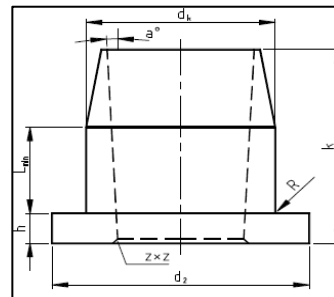
KAULUS
