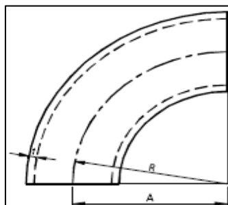
KÄYRÄ 90°
