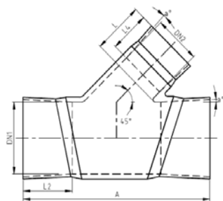
VEN T-KAPPALE 45° PN 6 LAMINOITU LIITOS
