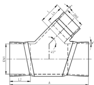
VE T-KAPPALE 45° PN 10 LAMINOITU LIITOS
