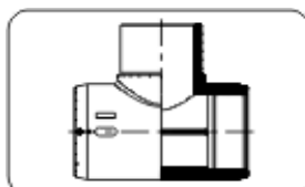
PEH SÄHKÖMUHVI T- HAARA
